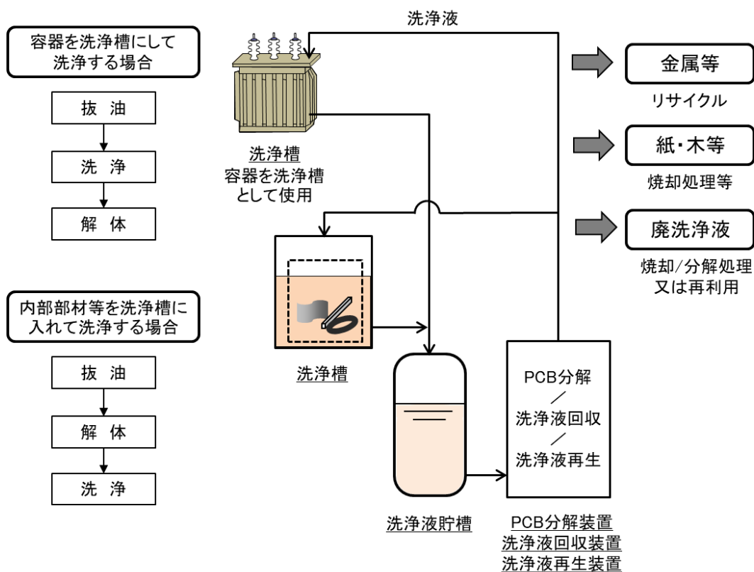
P C B に汚染された絶縁油を含む電気機器等の洗浄施設の例
